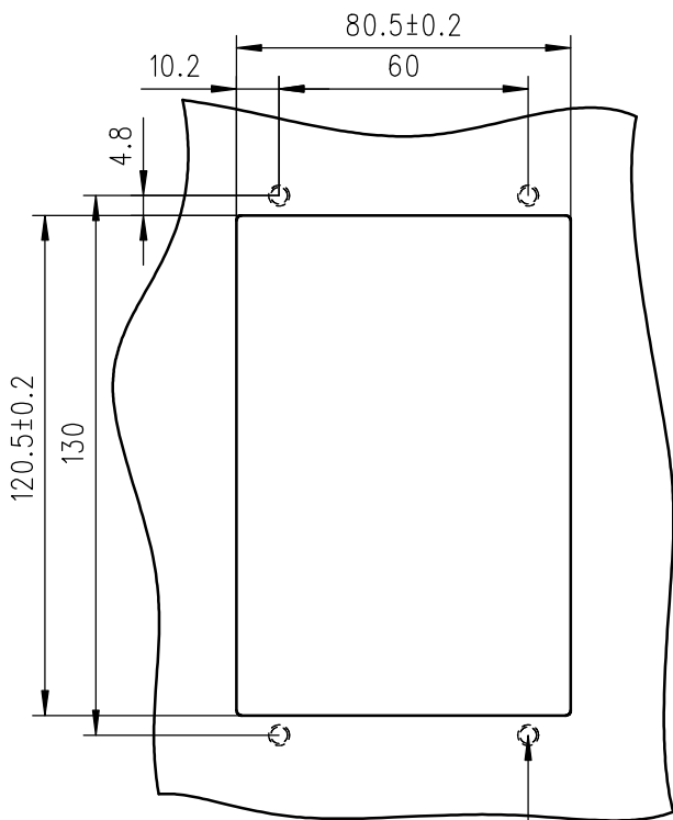
Schweissbolzen M5 (4x) AUSSCHNITT GERÄTEFRONT
